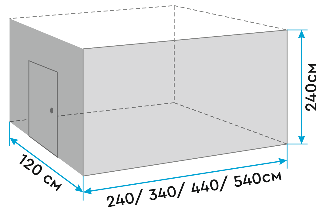
Стенд из бруса, обтянутый баннерной тканью
